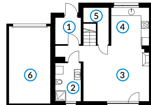
Rzut parteru
