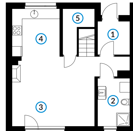
Rzut parteru
